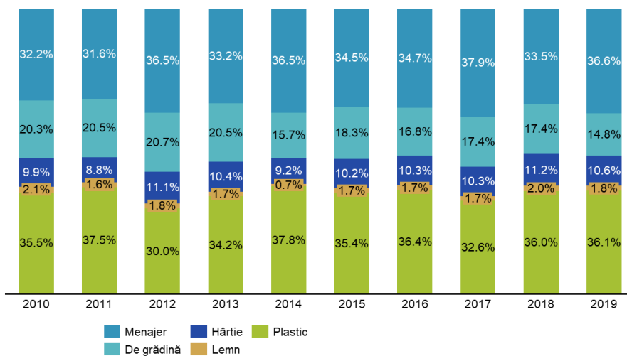
Figura 114. Compoziția deșeurilor
